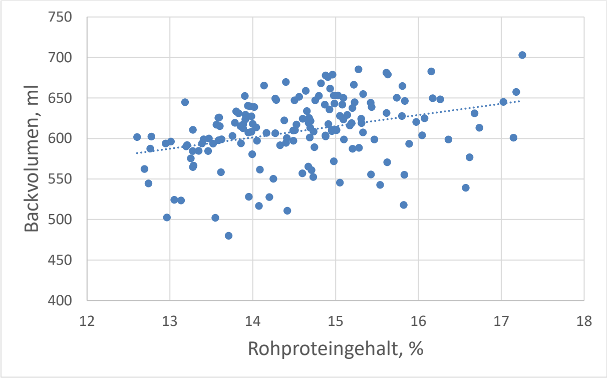
Fig. 2: Mittlere Backvolumen in Relation zum Rohproteingehalt bei 160 Dinkelsorten (gemittelt über drei Anbauorte) und der Pearson'sche Korrelationskoeffizient r = 0,34 .
